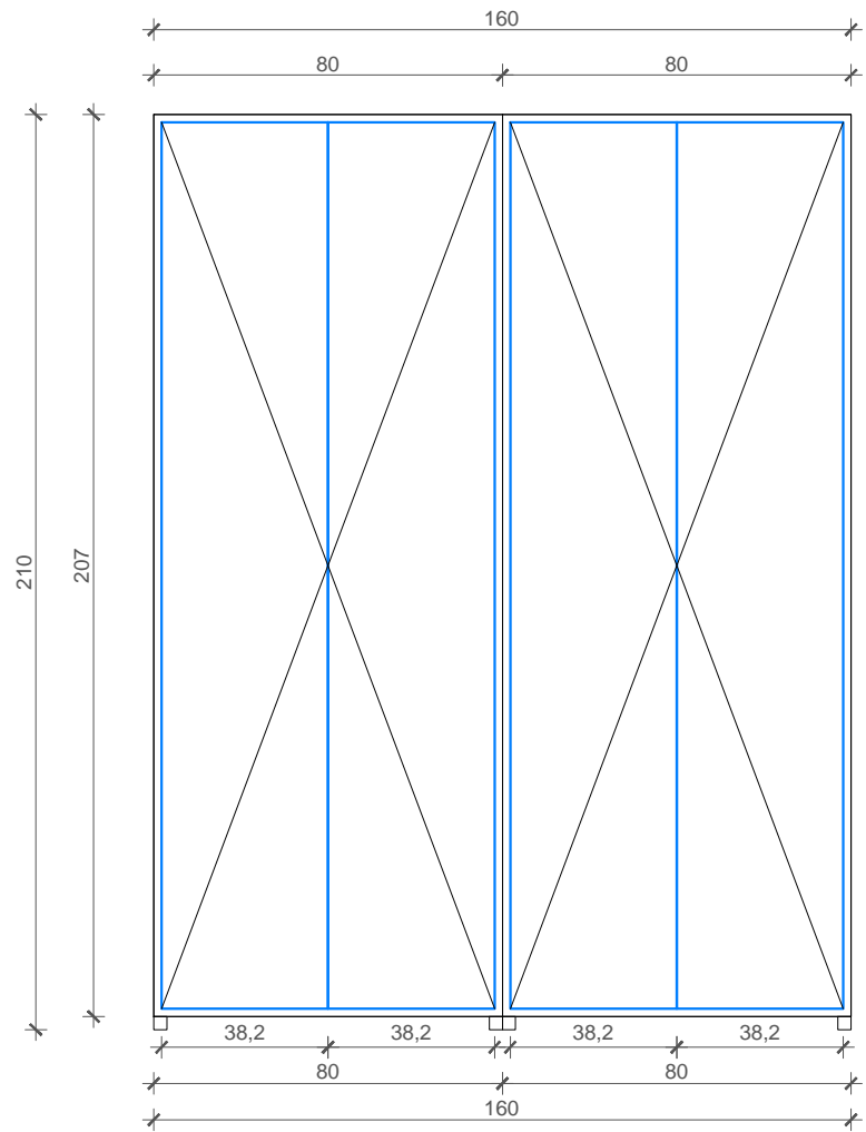
IZGLED IV otvaranje
